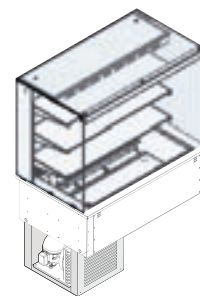
Umluft-Kühlvitrine mit 3 Etagen Vorhang Seite Kunde, Höhe: 1610 mm
