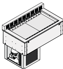
Gekühlte schale mit hinterem diffusor Höhe: 910 mm
