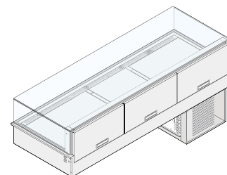
Abmaße (BxTxH): 1888 x 680 x 840 mm Bestell-Nr.: 70 VRJ 2C Preis: 8.677,00 €
